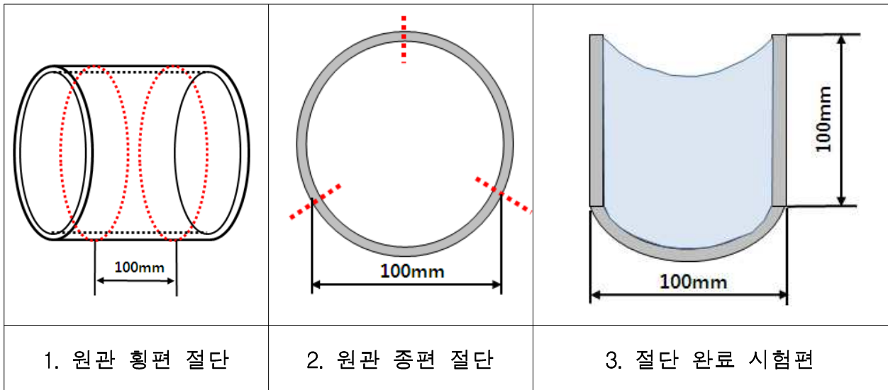
[그림2] 시험편 채취 방법1
